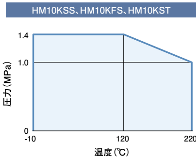
圧力 — 温度レーティング
