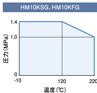
圧力 — 温度レーティング
