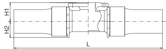
浅層埋設形
