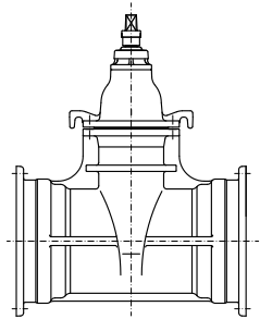
両受形
