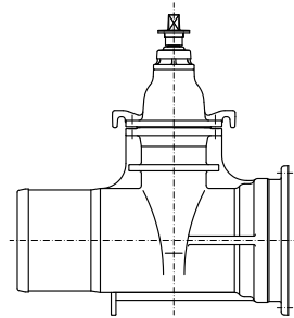
受挿し形
