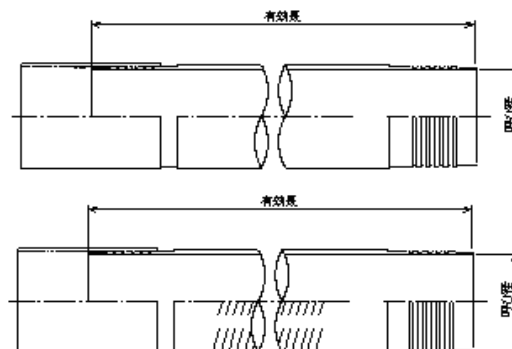
構造図
